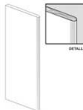
8 CANTO REDONDEADO PARA PUERTA VAIVÉN
