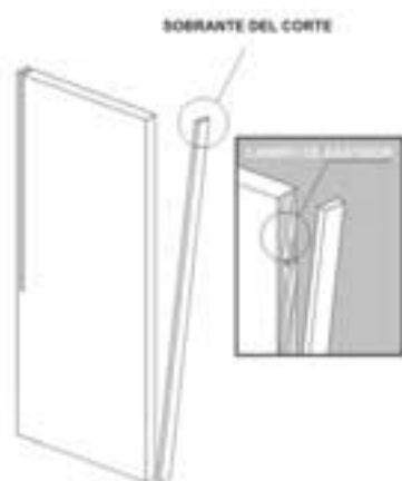
5 CORTE DE PUERTA CON CAMBIO DE BASTIDOR
